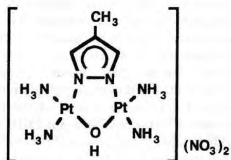
1,2-μH-Am-4mpz (Complex II)
